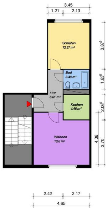
2-Raum - WE - WBS-70-Typ C1-rechts-
