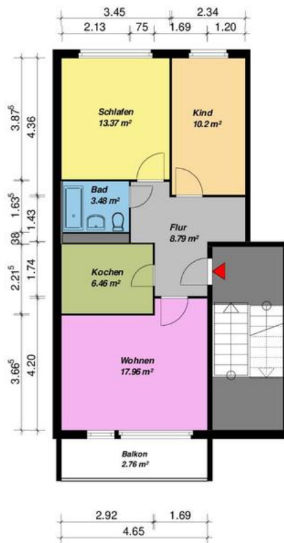
3-Raum -WE - WBS-70-Typ C1-links-mit Balkon
