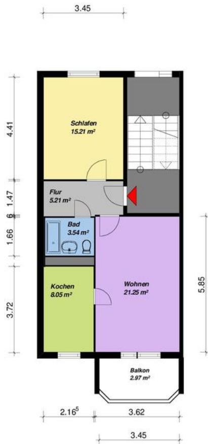
2-Raum-Wohnung- WBS 70, Typ C6.8 mit Balkon
