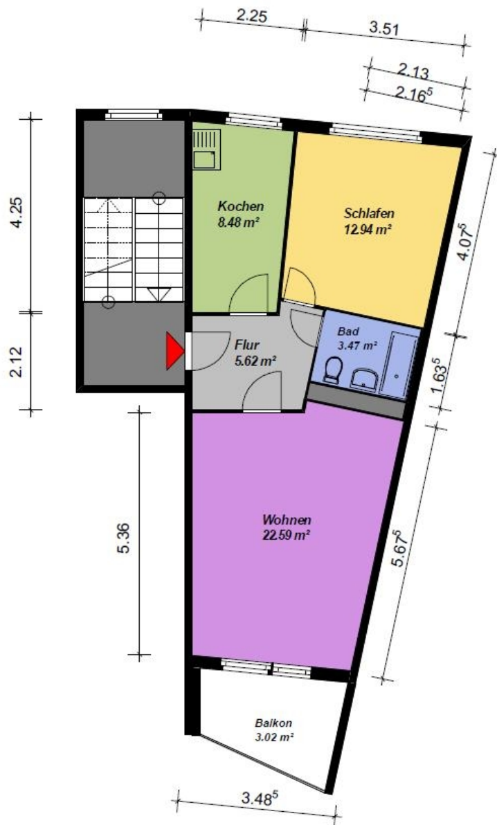
2 Raum-Wohnung, WBS 70, Typ HH, Segment A- Keil-mit Balkon
