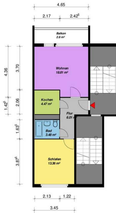
2-Raum -WE - WBS-70-Typ C1- rechts -EG-mit Balkon
