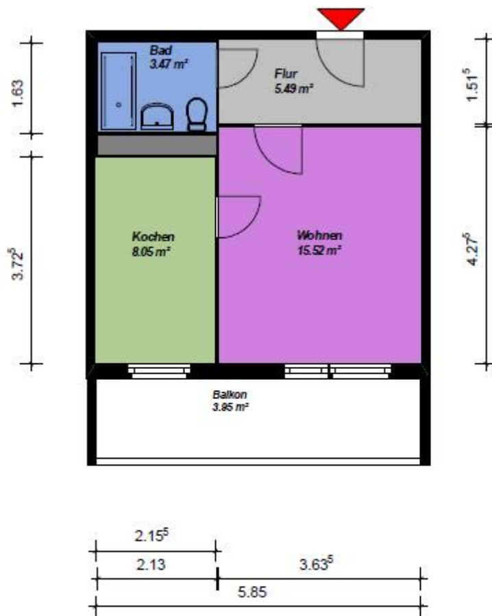
1 Raum-Wohnung, WBS 70, Typ HH, Segment A- ( 1.4.7.+10. Etage ) mit Balkon
