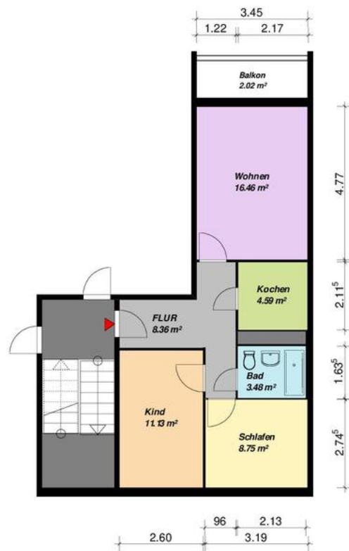
3 -Raum -WE - WBS-70-Typ C11- mit Balkon
