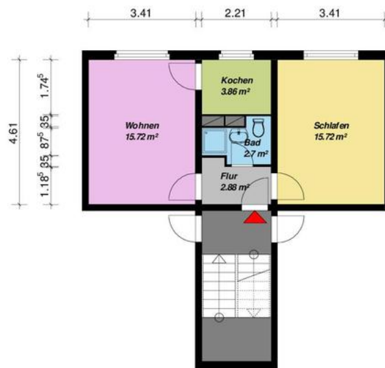
2-Raum-WE- Typ Brandenburg- Mittelwohnung-
